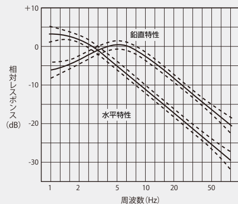
平たん特性の基準レスポンス及び許容差
