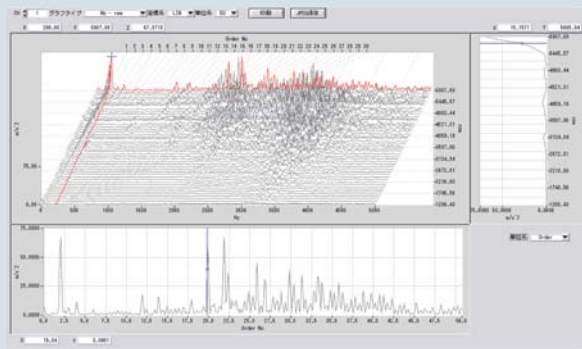
次数-レベル-回転数(ウォーターフォール図)
